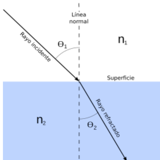
Figura 1. Esquema de la refracción de la luz.
