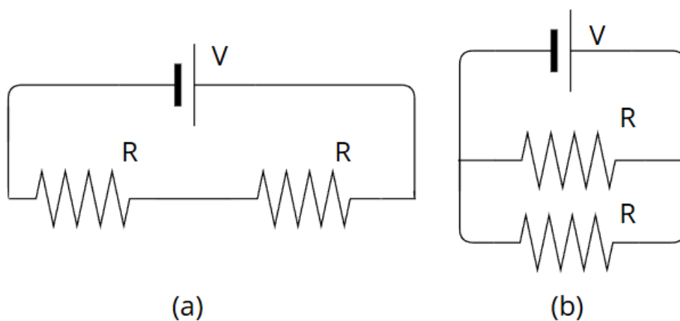
Figura 2. Esquema del circuito: (a) para el caso de las resistencias en serie y (b) para el caso de las resistencias en paralelo.
