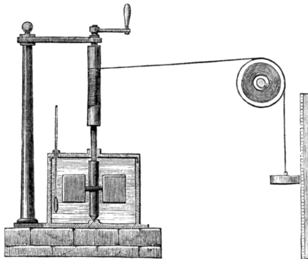
Figura 3. Representación del experimento de Joule.
