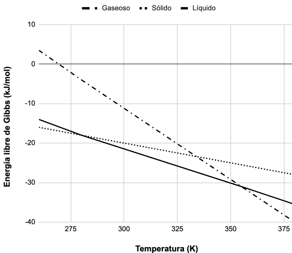
Gráfico 1. Comportamiento de la energía libre de Gibbs en las fases gaseosa, sólida y líquida del benceno en condiciones normales de presión.
