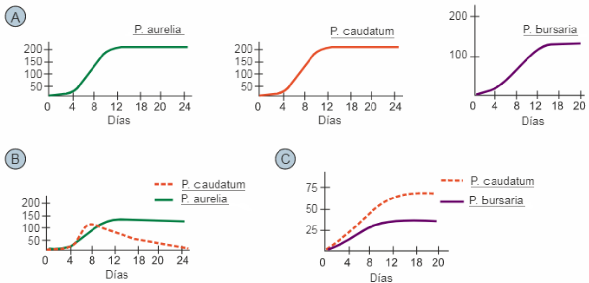
Figura 4. (A) Crecimiento de P. aurelia , P. caudatum , P. bursaria en forma aislada. (B) y (C) Crecimiento de P. aurelia , P. caudatum , P. bursaria en forma asociada.
