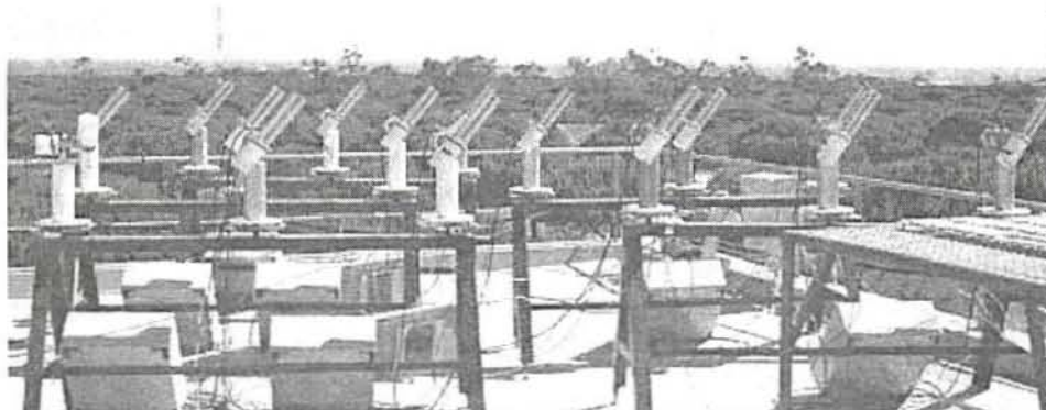
Figura 5. Intercomparación y calibración de instrumentos Cimel de la Red AERONET. (Campaña de verano, El Arenosillo 2006)
