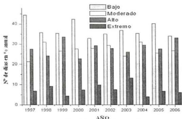
Figura 3. Índice de radiación solar ultravioleta en El Arenosillo. Estos datos se distribuyen diariamente a la Consejería de Medio Ambiente del Gobierno Andaluz para informar a la población. Se está trabajando actualmente en un modelo de predicción de UVB a nivel de Andalucía
