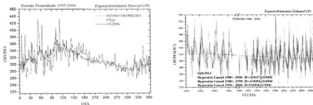
Figura 2. En el eje X aparecen representados los días del año desde el uno al 365, en el eje Y el contenido total de ozono en El Arenosillo
